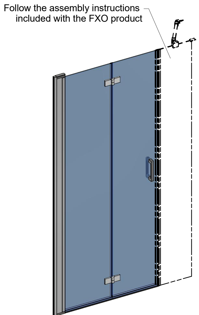
RIGHT Installation CI 2CL + CI FXO
