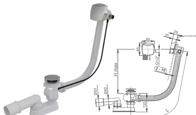
■ Sifons vannai ar uzpildi
