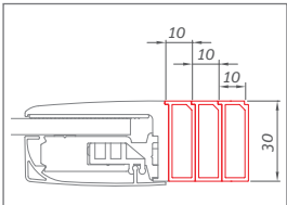
HITECH LINE celá série ELEGANT LINE celá série TOWER LINE modely: TR2, TDXX, TB
