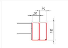
LEGA LINE modely: LLR2, LLS2, LLD01, LLD02, LLD2, LLB
